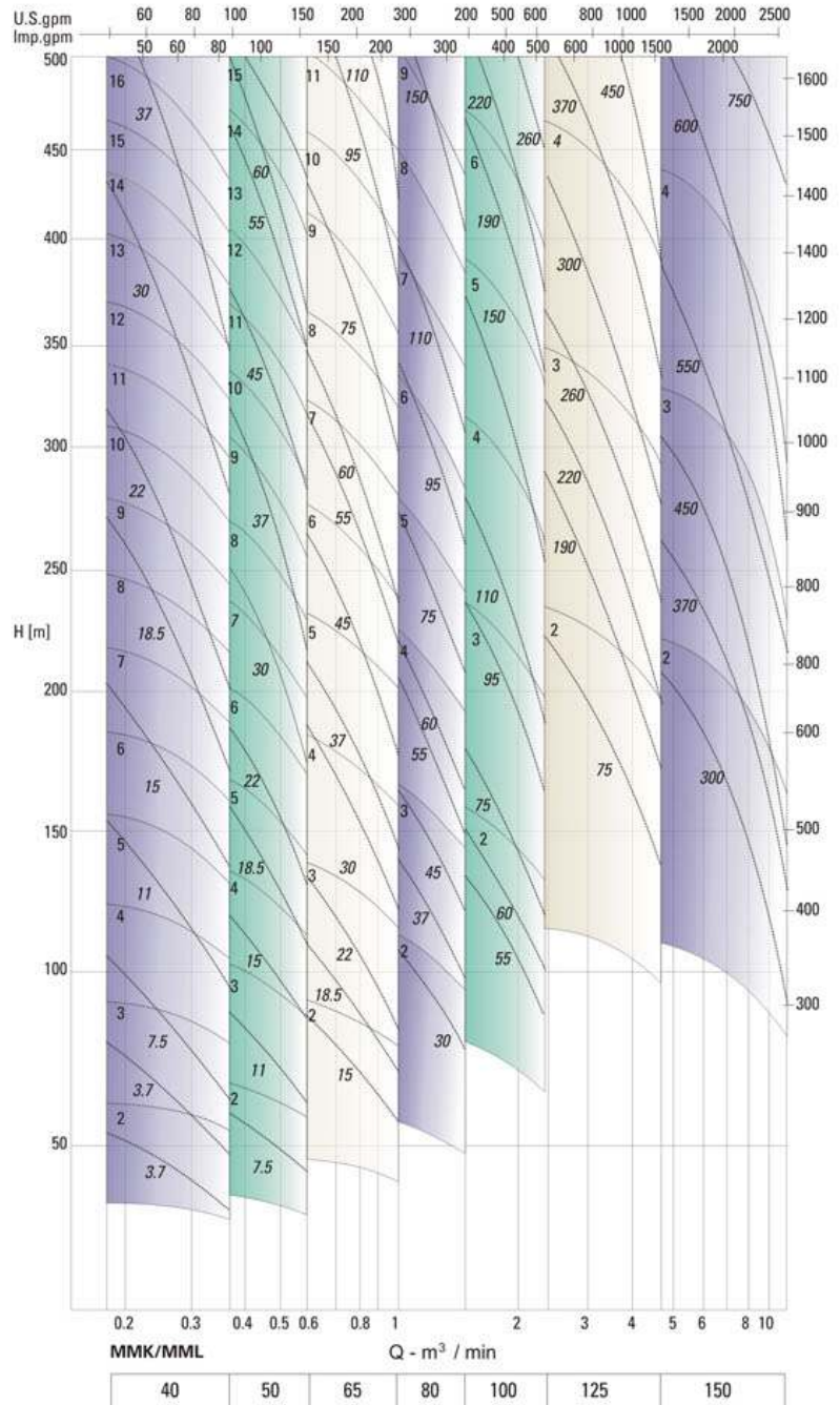
50Hz-2P (3000 r.p.m.)
