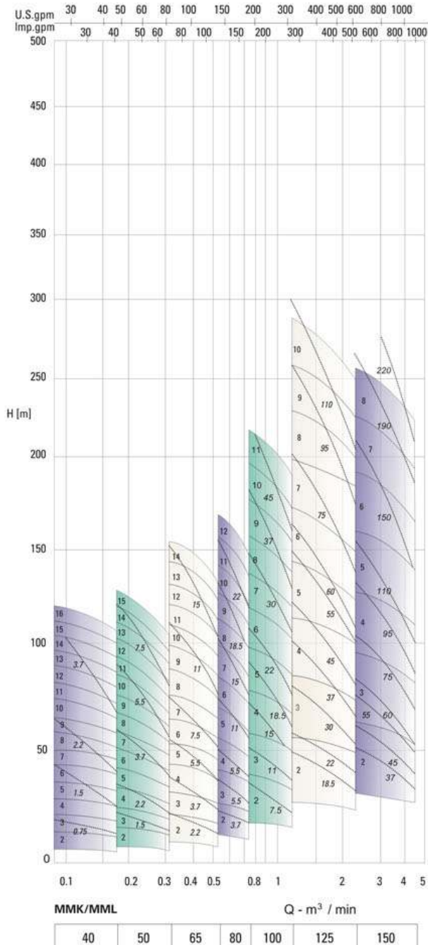
50Hz-4P (1500 r.p.m.)
